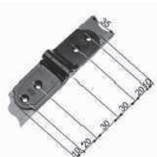
RUS11032 Bisagra plana Rústica placa vertical
