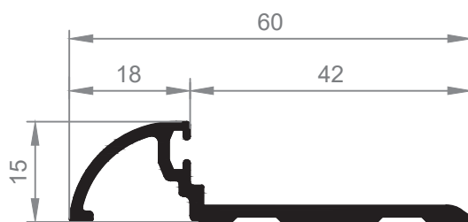
158 Perfil Suelo
