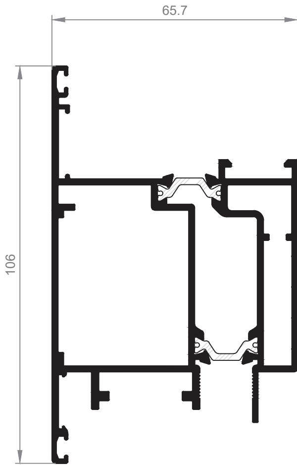
24628 Hoja "T" Apertura Exterior
