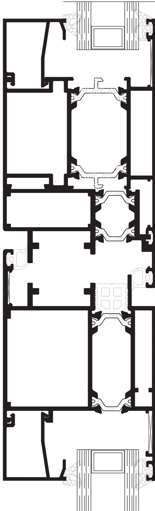
APERTURA INTERIOR
