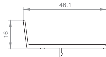
Sección
