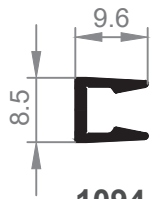
1094 Unión marcos con clip
