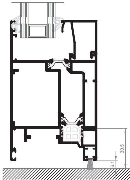
Variante sin pisadera
