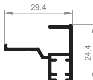
24642 Terminal Hoja puerta sin Pisadera
