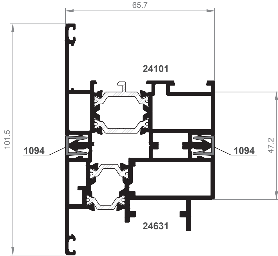
Unión marcos mediante clip ref. 1094
