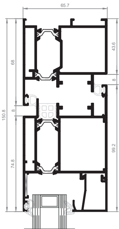
Sección A-B
