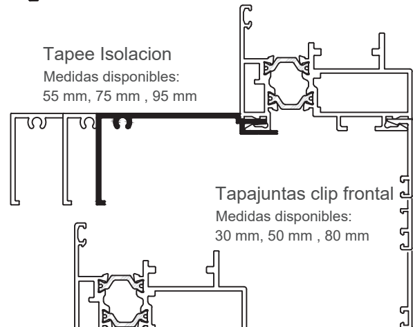
Tapajuntas
