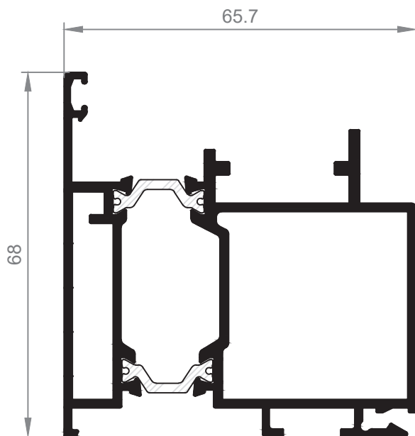
24671 Marco Clip Interior puerta
