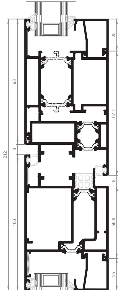
Sección B-C
