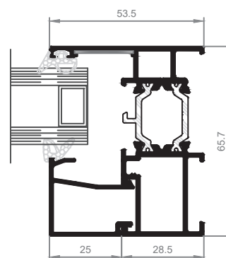
Detalle C
