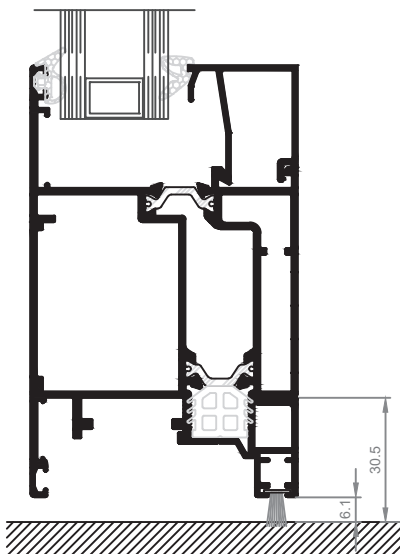
Sección C
