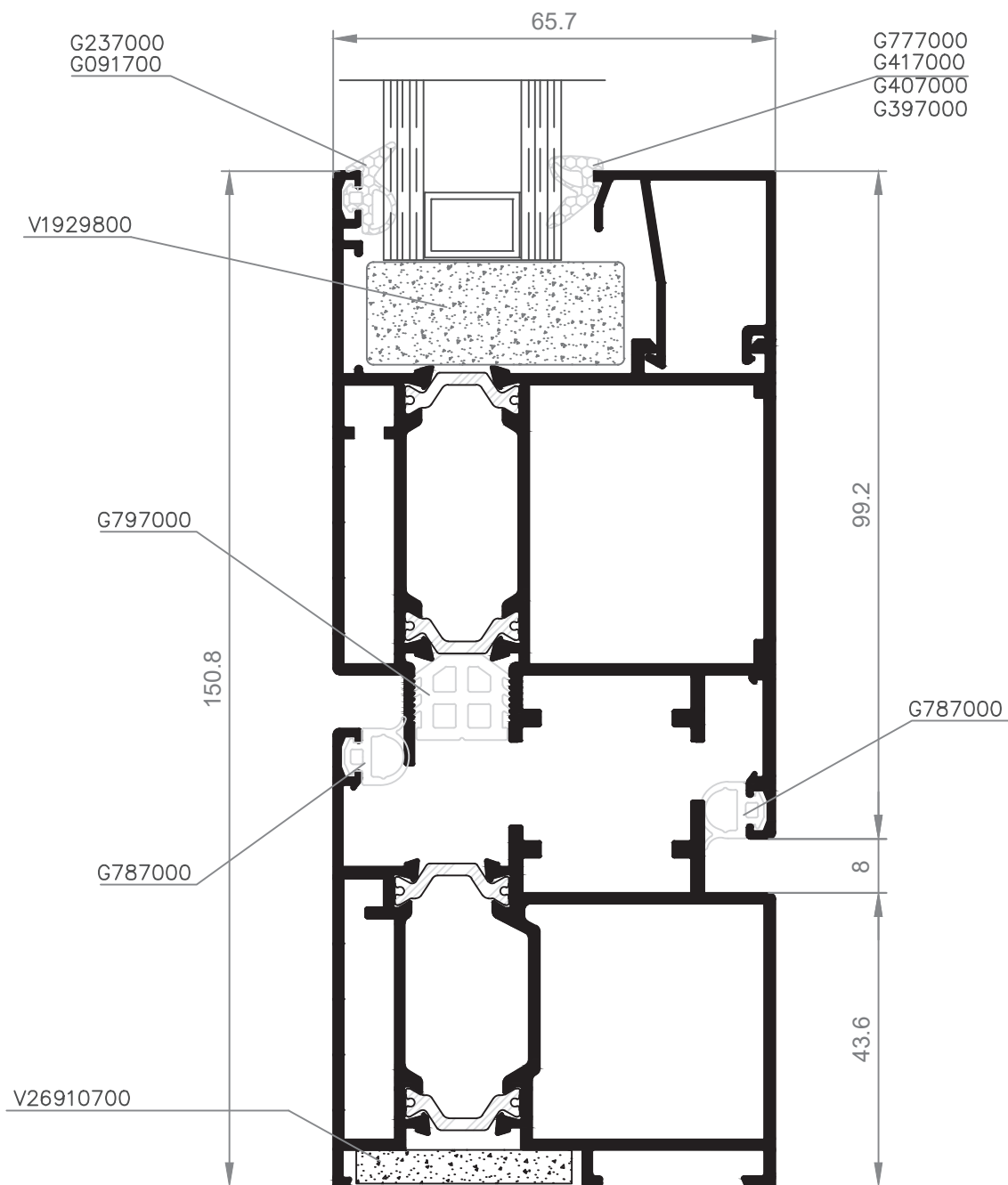
G787000 Junta batiente
