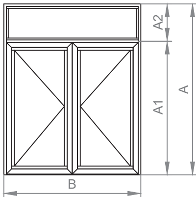
Puerta 2 Hojas+Fijo Superior Apertura Interior
