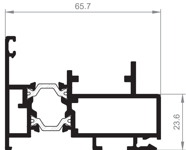
24651 Marco Clip Interior puerta reducido
