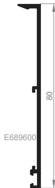
346 Tapajuntas 80 mm. Clip Frontal
