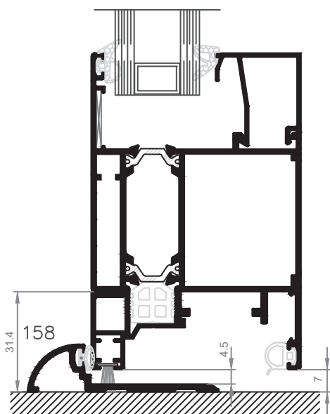
Variante sin pisadera
