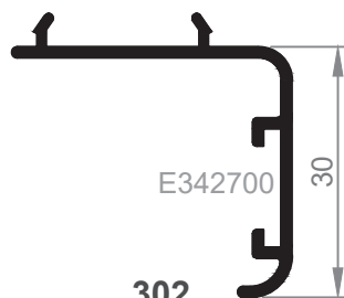
302 Tapajuntas Clipado
