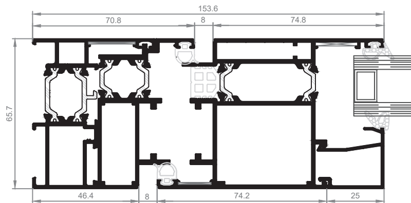
Detalle E
