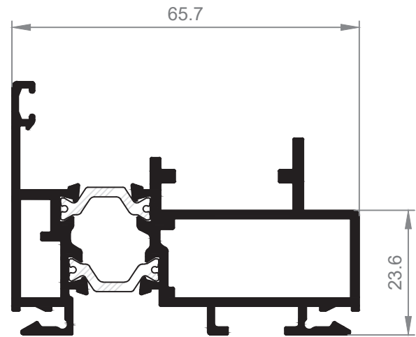
24631 Marco Clip puerta reducido
