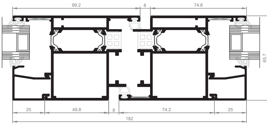
Detalle E
