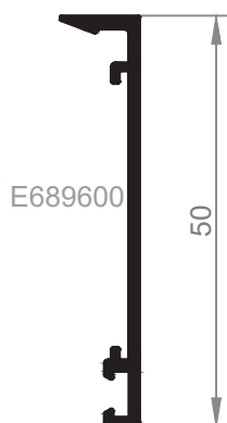
345 Tapajuntas 50 mm. Clip Frontal
