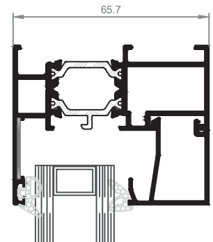
Sección A-B
