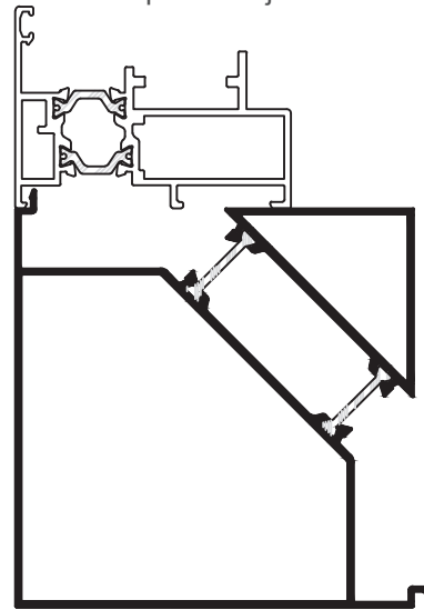
Esquinero Fijo
