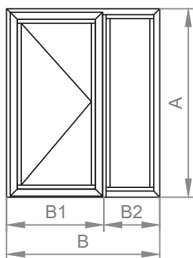
Puerta 1 Hoja+Fijo Lateral Apertura Interior
