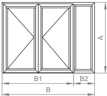
Puerta 2 Hojas+Fijo Lateral Apertura Interior
