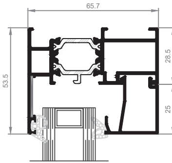
Sección A
