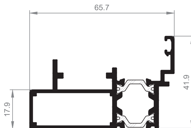
24623 INVERSOR Apertura Interior 2 hojas Suministro de material a 4500mm.
