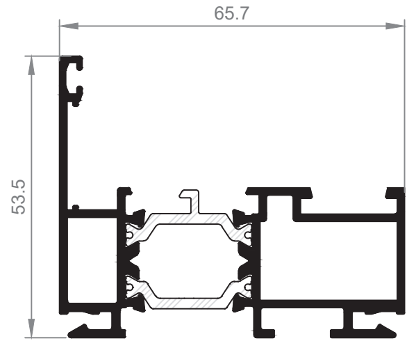
24101 Marco Clip Frontal
