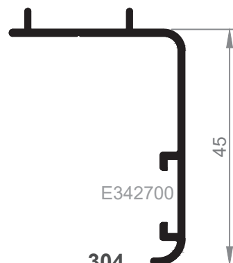
304 Tapajuntas Clipado
