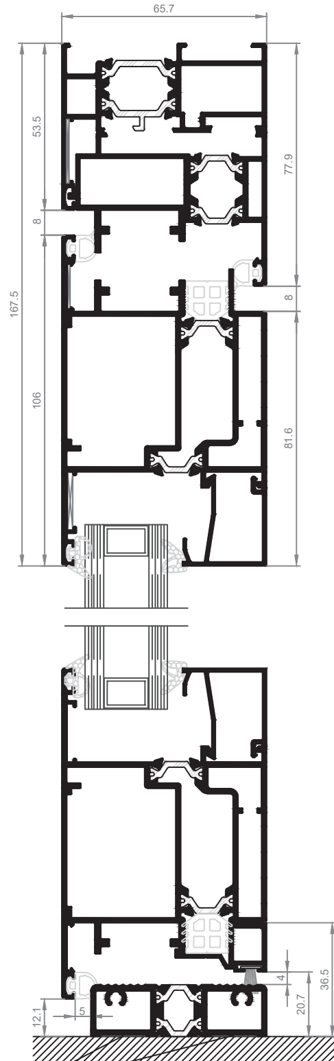
Sección A-B
