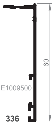
336 Tapajuntas 60
