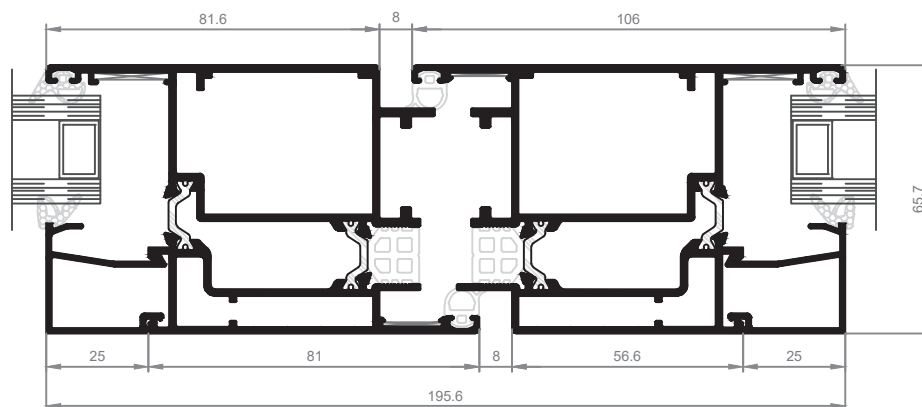
Detalle E
