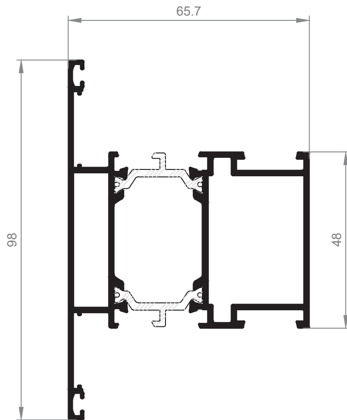
24023 Travesaño
