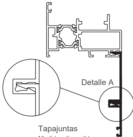
Tapa interior guía clip
