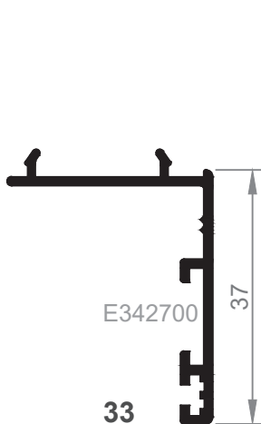
33 Tapajuntas 37 Clipado
