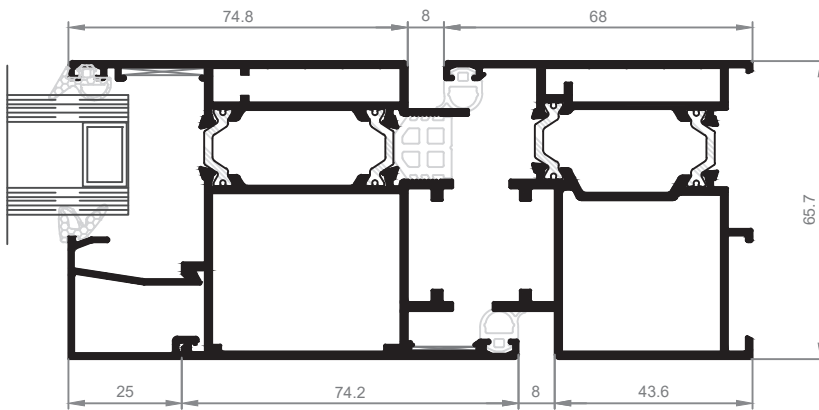
Detalle C
