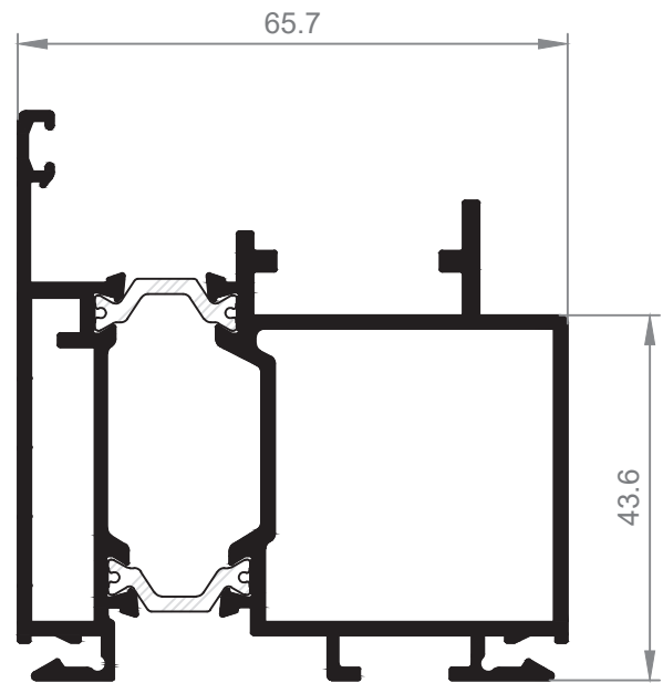
24661 Marco Clip puerta
