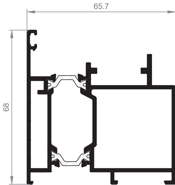
24621 Marco puerta
