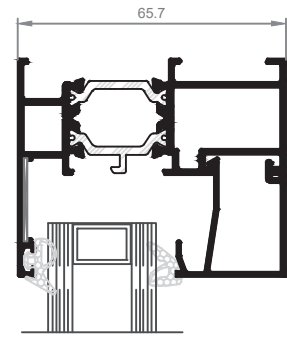
Sección A-B
