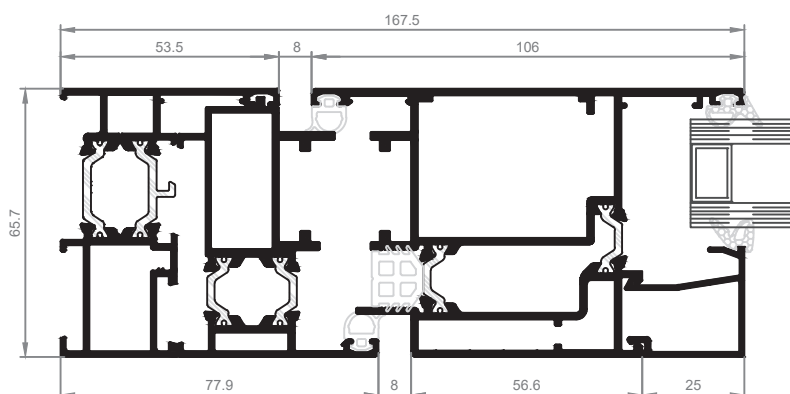
Detalle E
