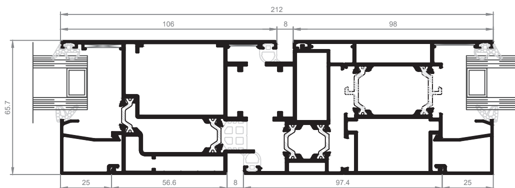
Detalle F
