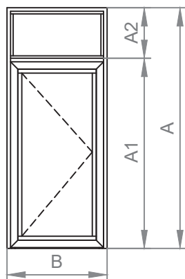
Puerta 1 Hoja+Fijo Superior Apertura Exterior
