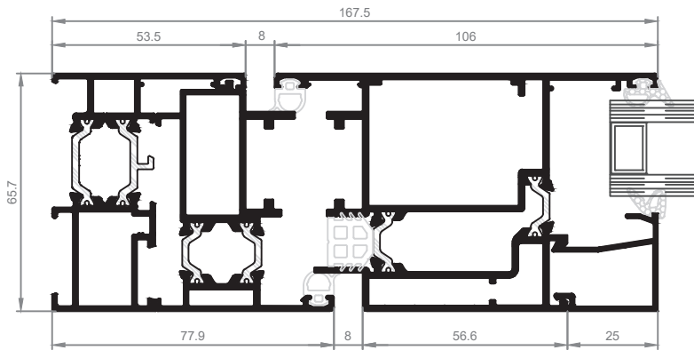
Sección D
