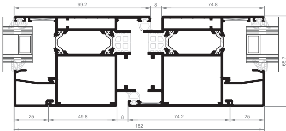
Detalle F
