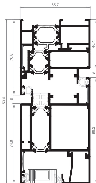
Sección A-B
