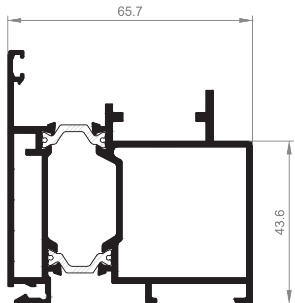
24681 Marco Clip Exterior puerta
