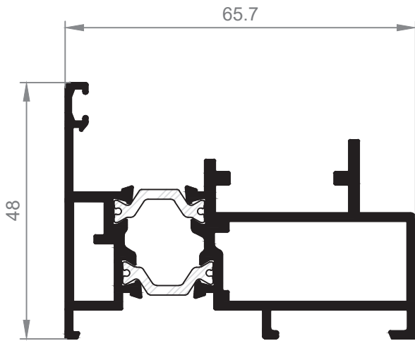
24601 Marco puerta reducido
