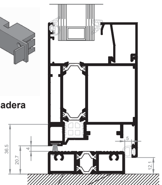
Cama de silicona
