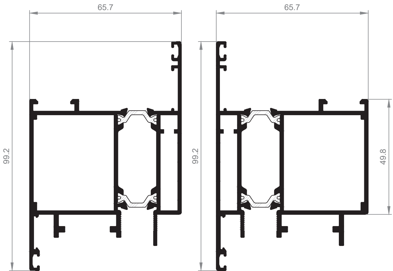
24622 Hoja "Z" Apertura Interior
