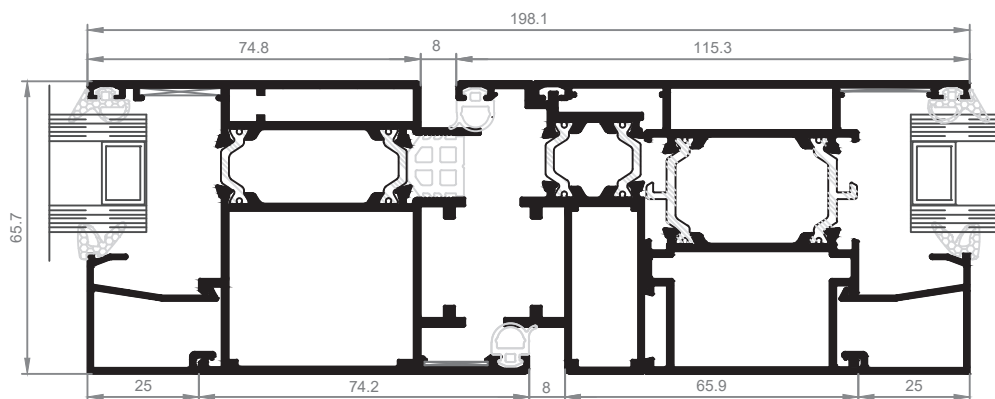
Detalle F
