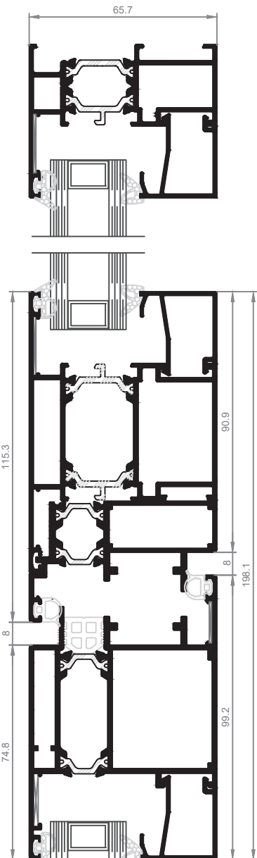
Sección A-B-C
