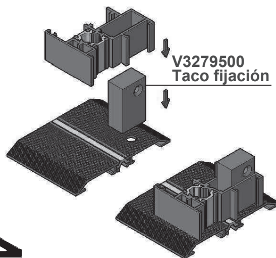
Montaje ref. 24159
