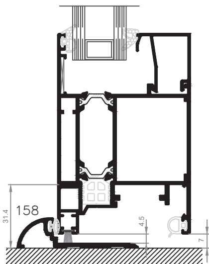
Variante sin pisadera
