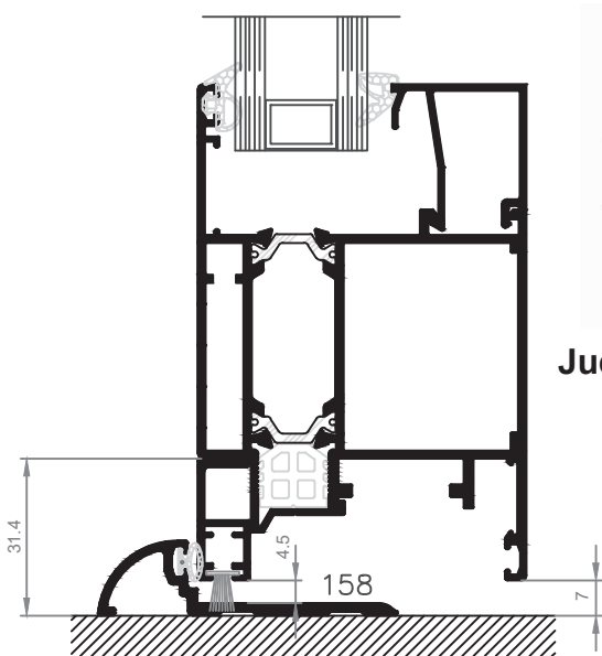
VARIANTE SIN PISADERA
