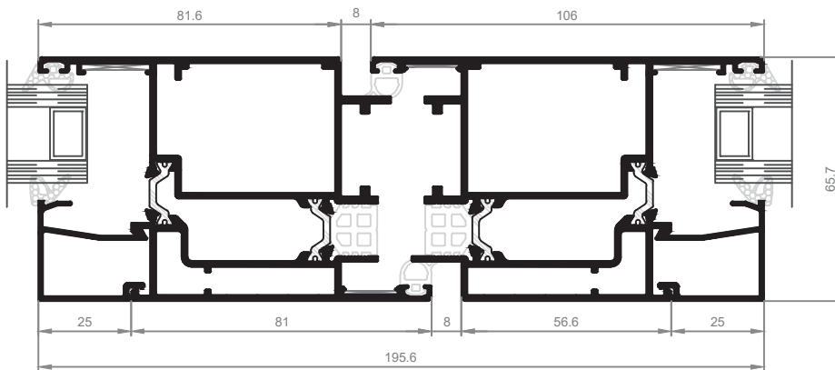
Detalle D
