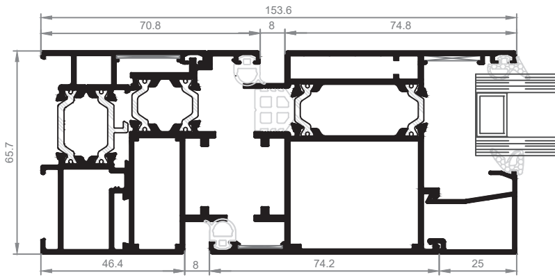
Detalle E
