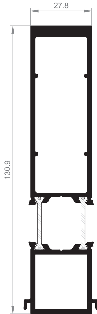
24112 Union RT Refuerzo
