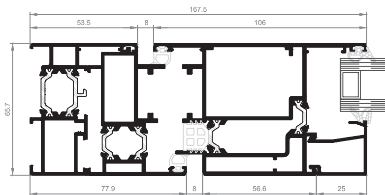
Detalle E
