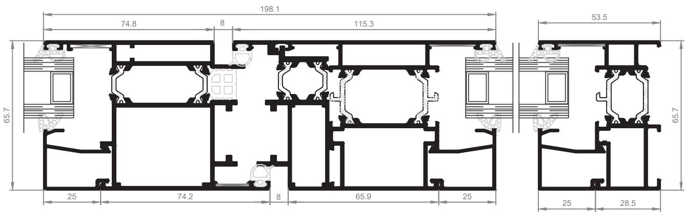
Detalle C-D
