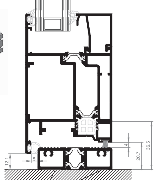
Juego tapones pisadera (opcional) TP6910802
