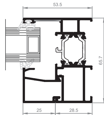
Detalle C
