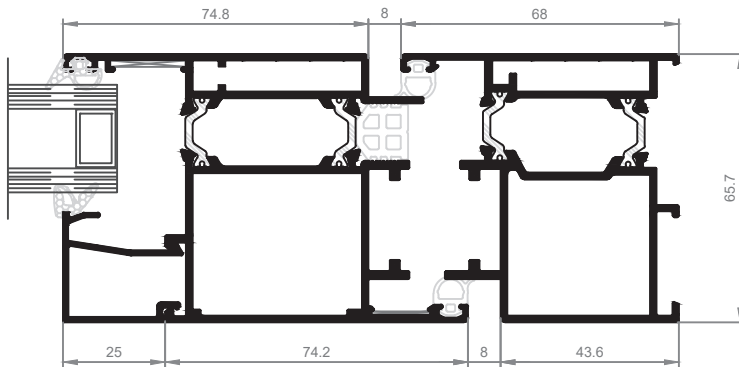
Detalle C
