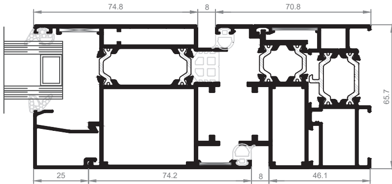
Detalle C
