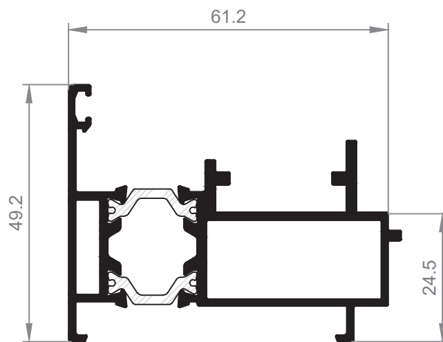
24650 Conversor Apertura Exterior
