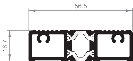
24658 Pisadera rotura Platinum 66
