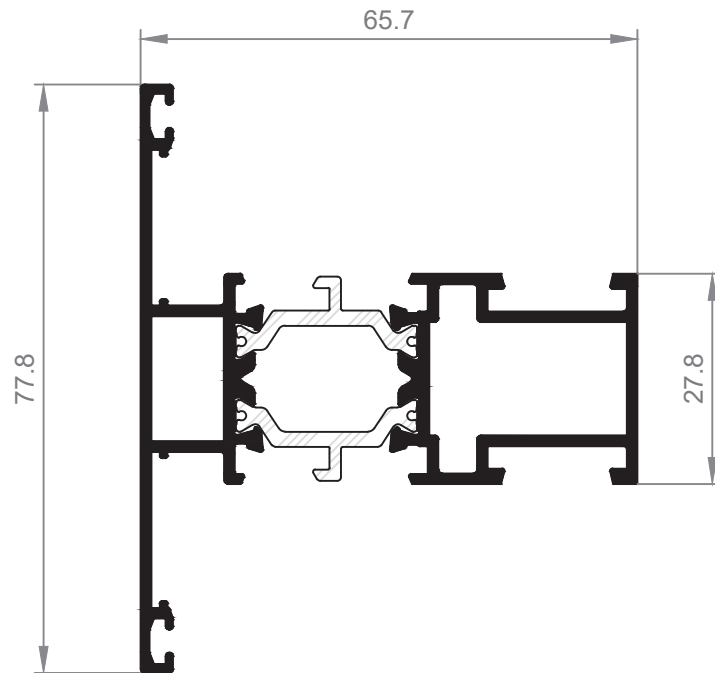
24003 Travesaño
