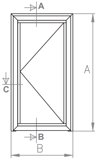
Puerta 1 Hoja Apertura Interior
