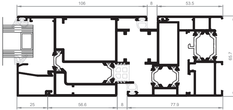
Detalle D
