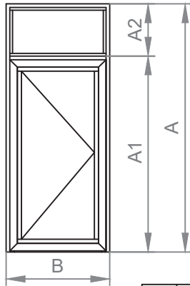
Puerta 1 Hoja+Fijo Superior Apertura Interior
