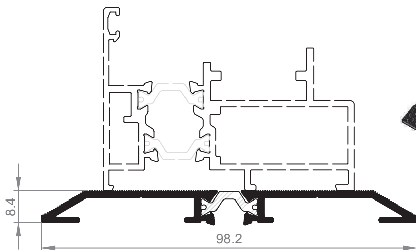
24159 Pisadera Rotura 8.4x98mm.
