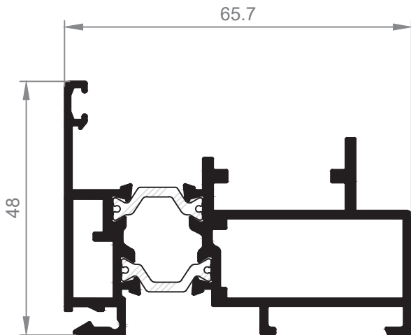
24641 Marco Clip Exterior puerta reducido
