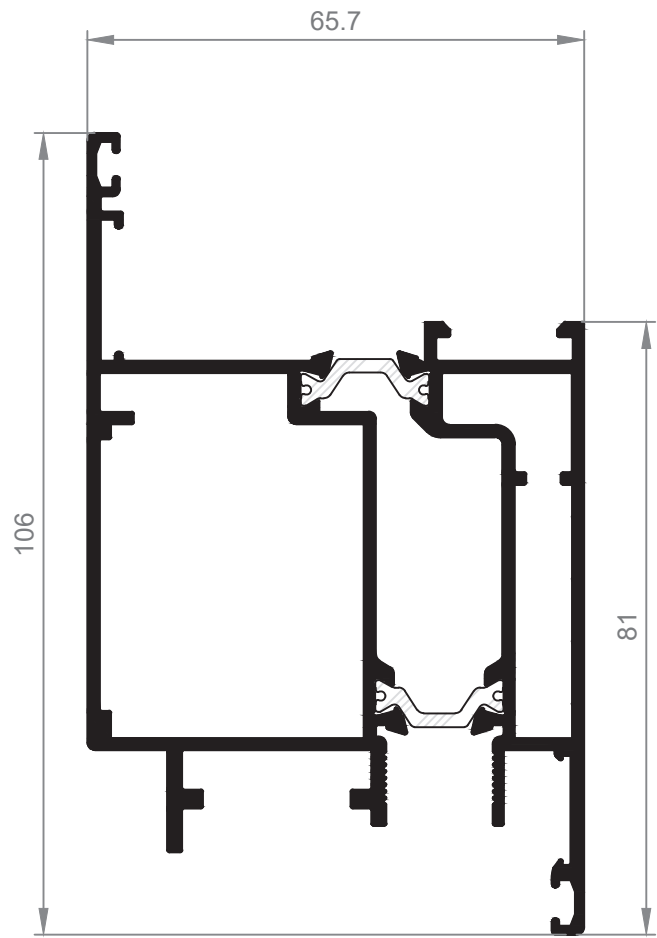
24629 INVERSOR Apertura Exterior 2 hojas Suministro de material a 4500mm.
