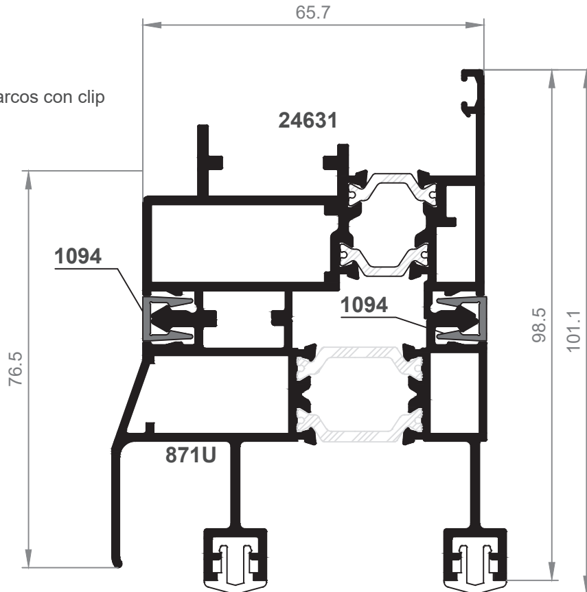
Unión marcos ref. 24631 y 871U mediante clip ref. 1094
