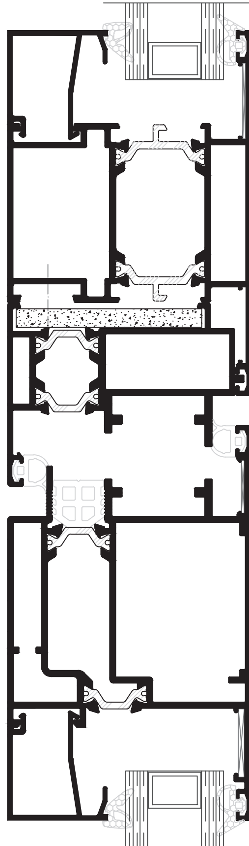
APERTURA EXTERIOR
