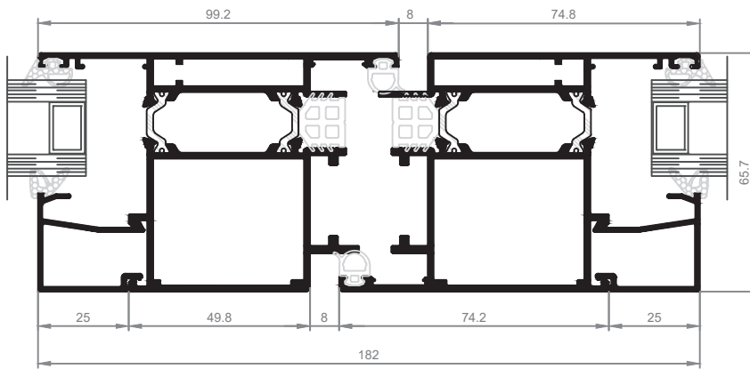
Detalle D
