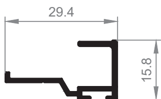
24643 Terminal Hoja puerta con Pisadera
