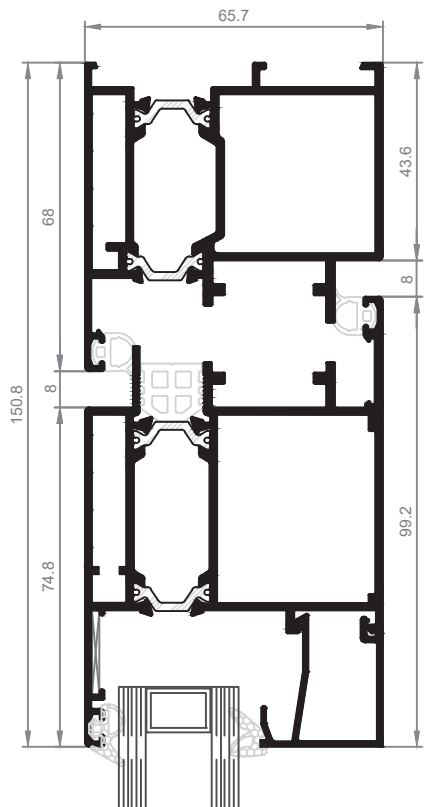
Sección A-B
