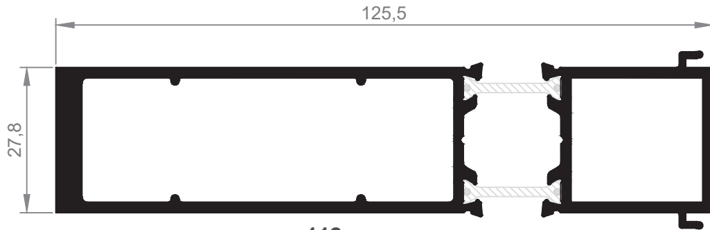
112 Union RT Refuerzo
