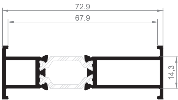
8720 Unión Marcos 870 CR
