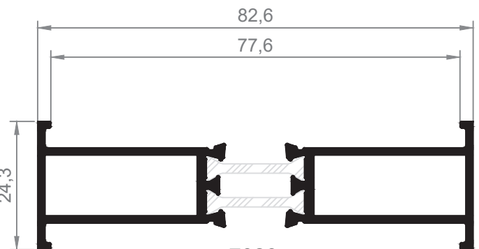
7020 Unión Marcos 77 RT
