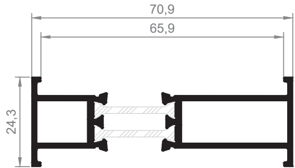
24000 Unión Marcos Serie 24000 RT
