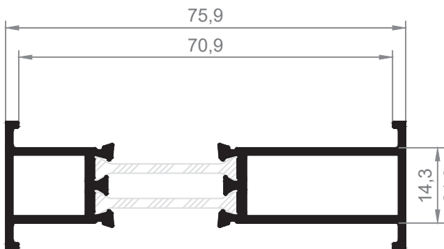
820 Unión Marcos 70 RT
