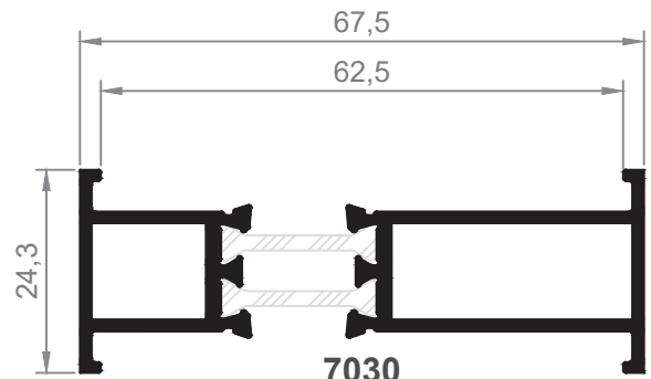
7030 Unión Marcos 62 RT
