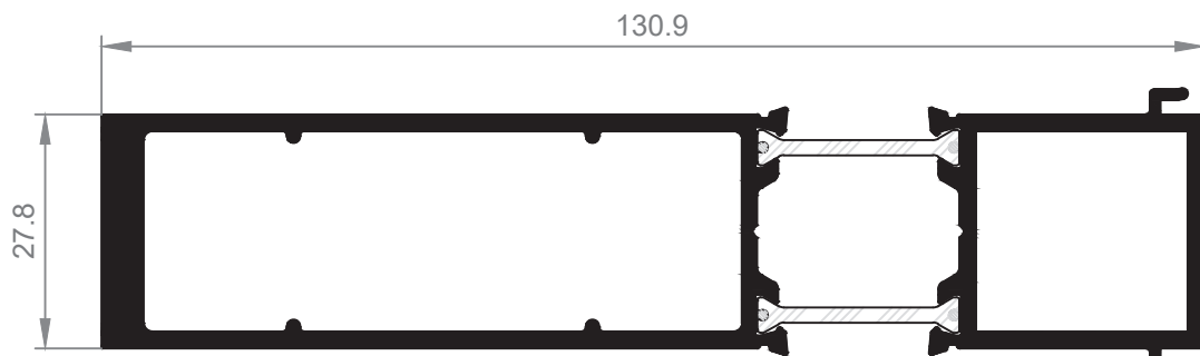
24112 Union RT Refuerzo
