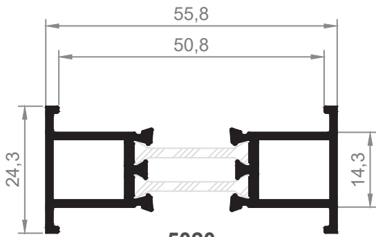
5020 Unión Marcos 50 RT
