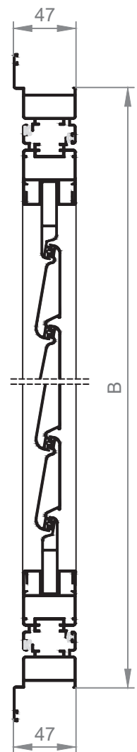
SECCION B-B'
