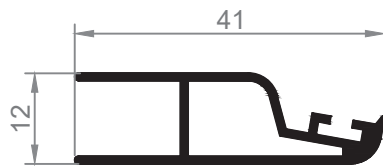
215G Lama media mallorquina *Consultar stock
