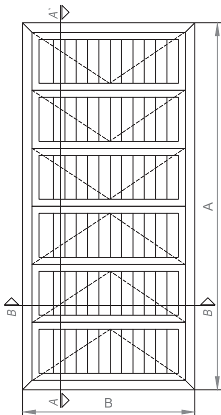
Contraventana practicable 6H perfil 214G
