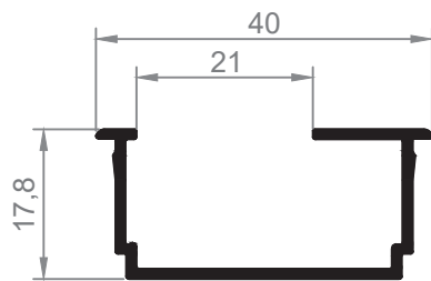
222 Suplemento de 21mm.
