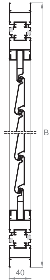
SECCION B-B'
