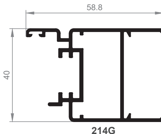
Marco hoja mallorquina
