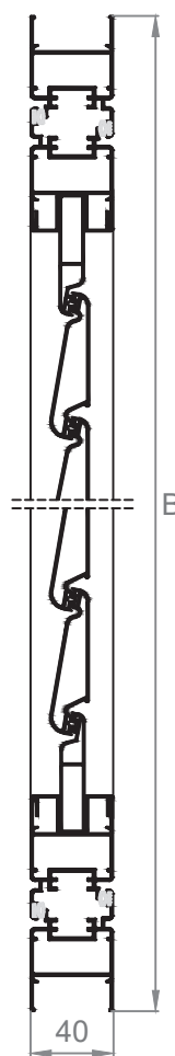
SECCION B-B'
